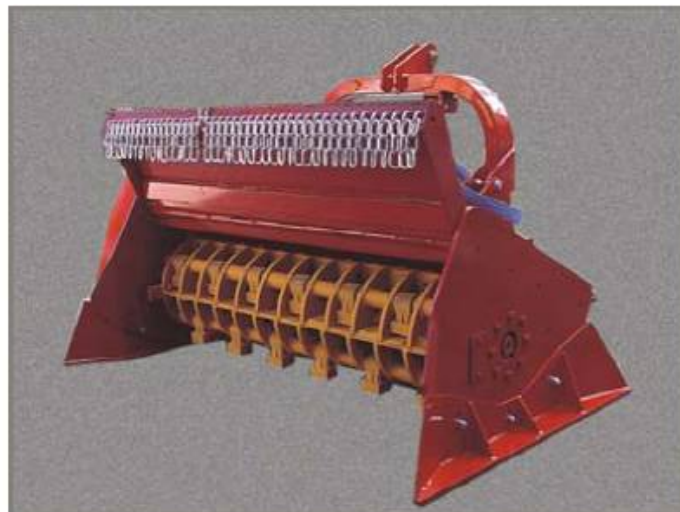
Rotor MIDIPIERRE. Masinile cu rotor mai mare de 175 cm sunt prevazute cu transmisie dubla. Toate utilajele au carcasa HARDOX.
